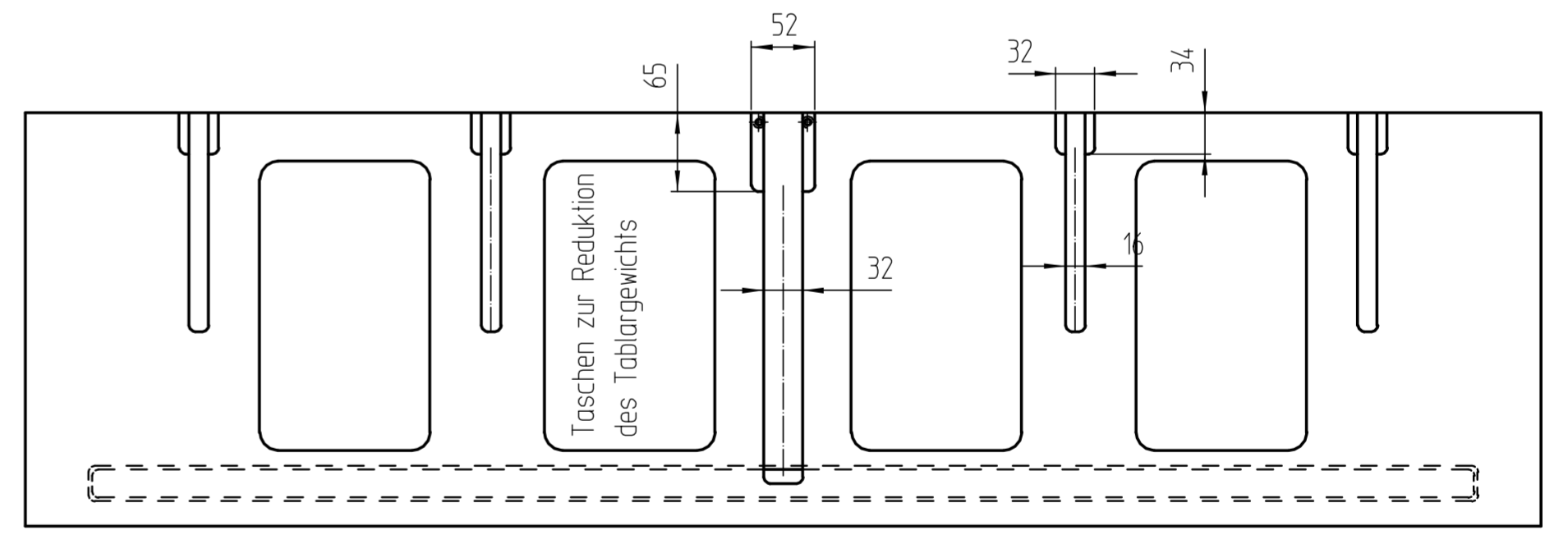
Innenansicht untere Schale
