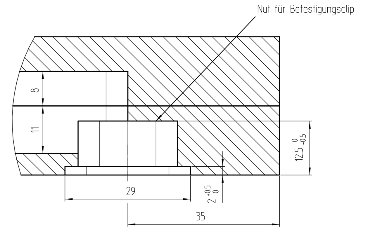
Innenansicht obere Schale
