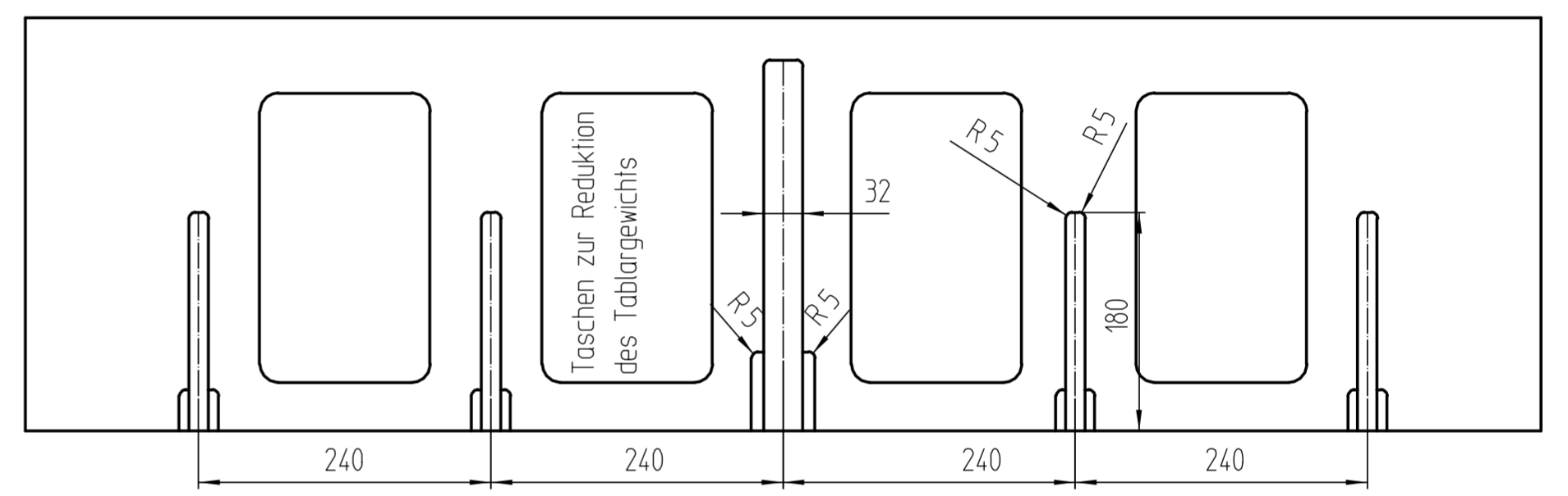
Innenansicht obere Schale
